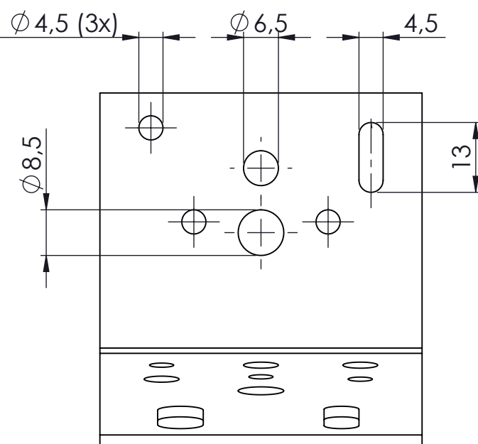
AANZICHT A
