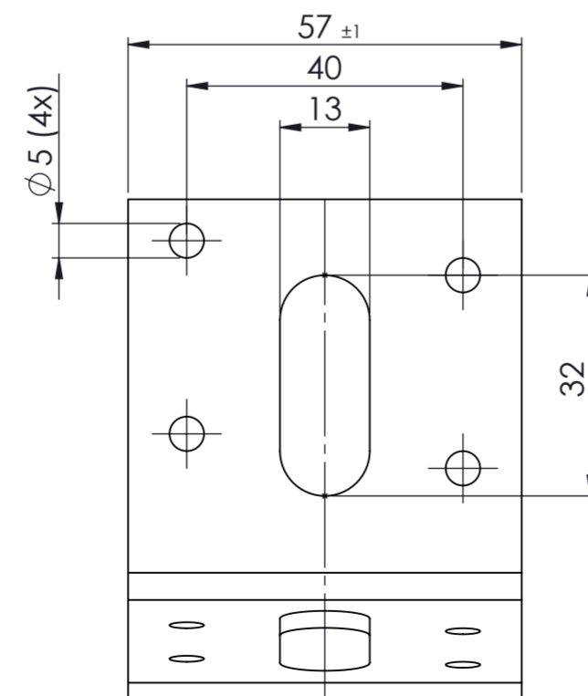
AANZICHT VOLGENS A
