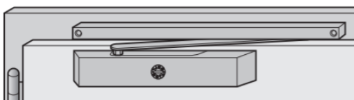
Deurbladmontage aan scharnierzijde T6 of T46
