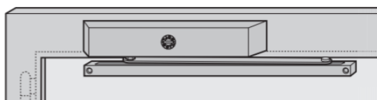
Kozijnmontage aan niet-scharnierzijde T6 of T46
