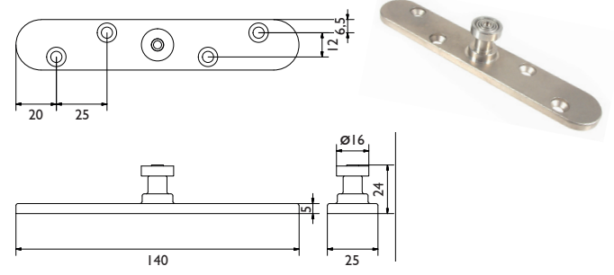
Geleider 106HSS/94
