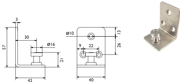
Geleider 102SS/94
