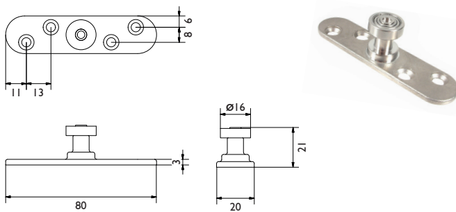
Geleider 106SS/94
